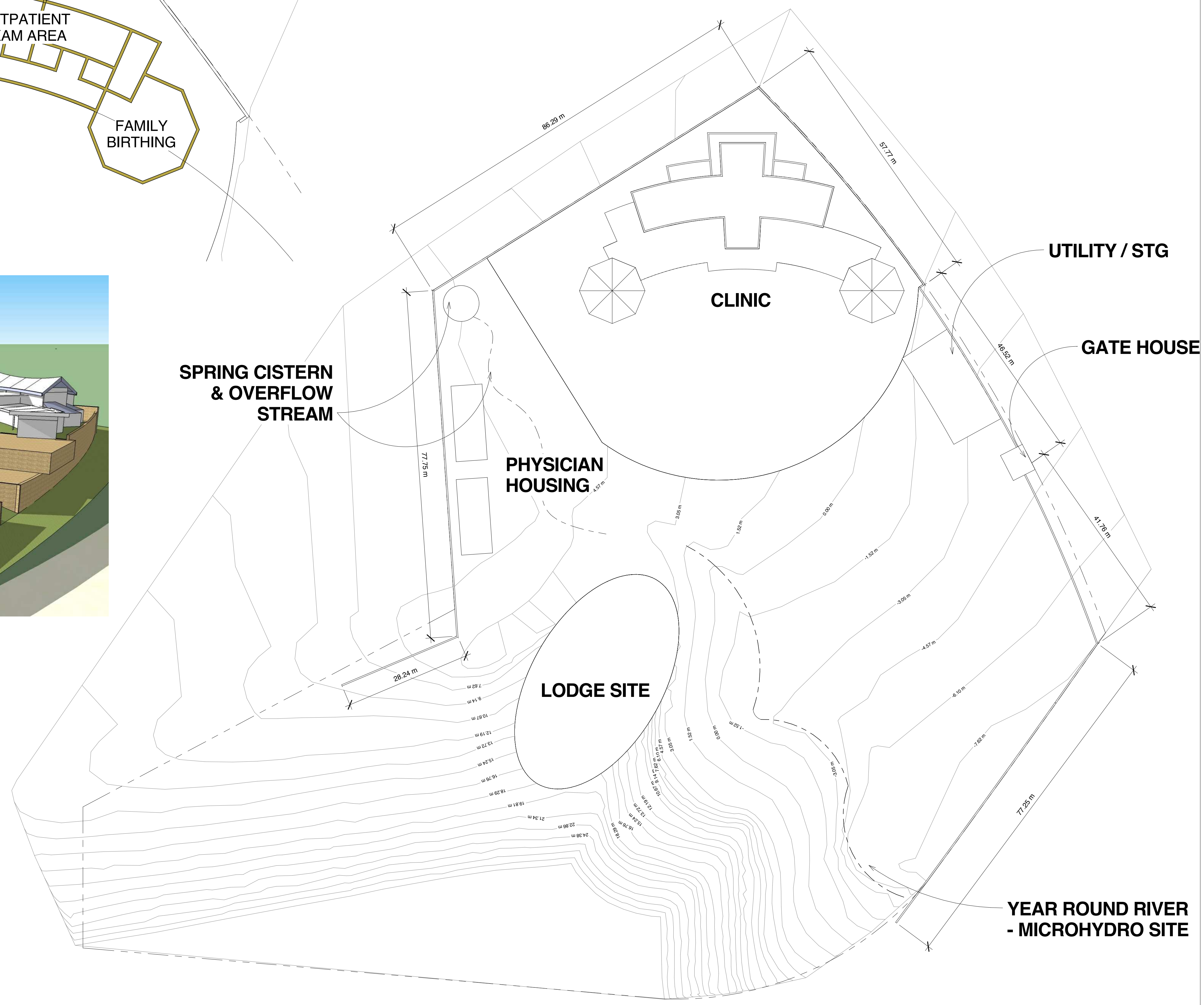
1 SITE PLAN 1:480
